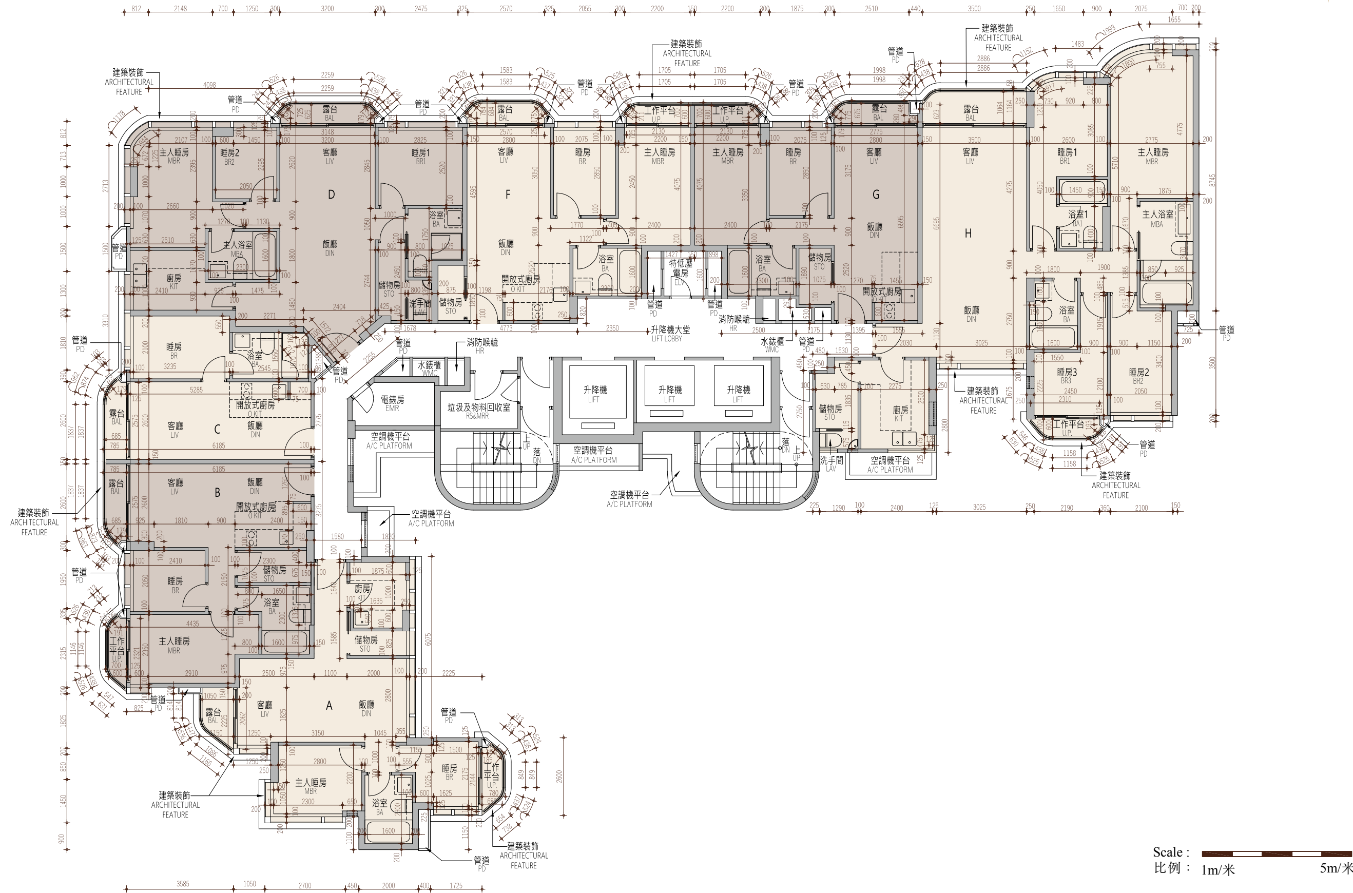
19/F Floor Plan 19樓 樓面平面圖
